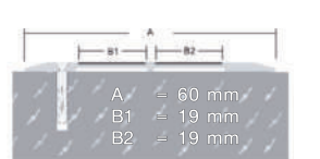
ASM-Profil TP 400-F
