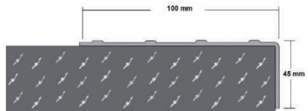
Sonderprofil aus V2 A Edelstahl, 1.4301 mit 4 Reihen Trittschutznocken Stärke 1,5 mm, Auflage 100 mm, Höhe 45 mm
