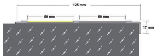
Sonderprofil aus V2 A Edelstahl, 1.4301 mit Trittschutznocken für 2 Kundeneinlagen Stärke 1,5 mm, Auflage 125 mm, Höhe 17 mm
