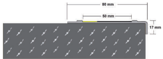
Sonderprofil aus V2 A Edelstahl, 1.4301 mit Trittschutznocken für Kundeneinlage Stärke 1,5 mm, Auflage 80 mm, Höhe 17 mm
