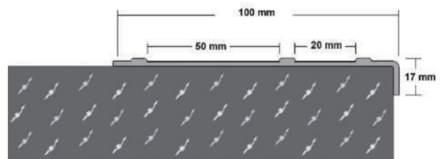
Sonderprofil aus V2 A Edelstahl, 1.4301 mit Trittschutznocken für 2 Kundeneinlagen Stärke 1,5 mm, Auflage 100 mm, Höhe 17 mm
