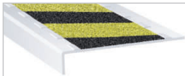
Sonderprofil aus V2 A Edelstahl, 1.4301 mit Trittschutznocken für Kundeneinlage Stärke 1,5 mm, Auflage 80 mm, Höhe 17 mm
