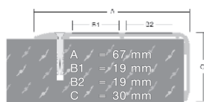
ASM-Profil TP 400
