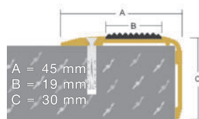
ASM-Profil TP 102
