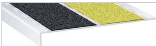
Sonderprofil aus V2 A Edelstahl, 1.4301 mit Trittschutznocken für 2 Kundeneinlagen Stärke 1,5 mm, Auflage 125 mm, Höhe 17 mm
