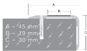
ASM-Profil TP 300
