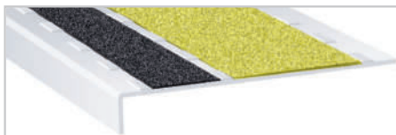
Sonderprofil aus V2 A Edelstahl, 1.4301 mit Trittschutznocken für 2 Kundeneinlagen Stärke 1,5 mm, Auflage 100 mm, Höhe 17 mm
